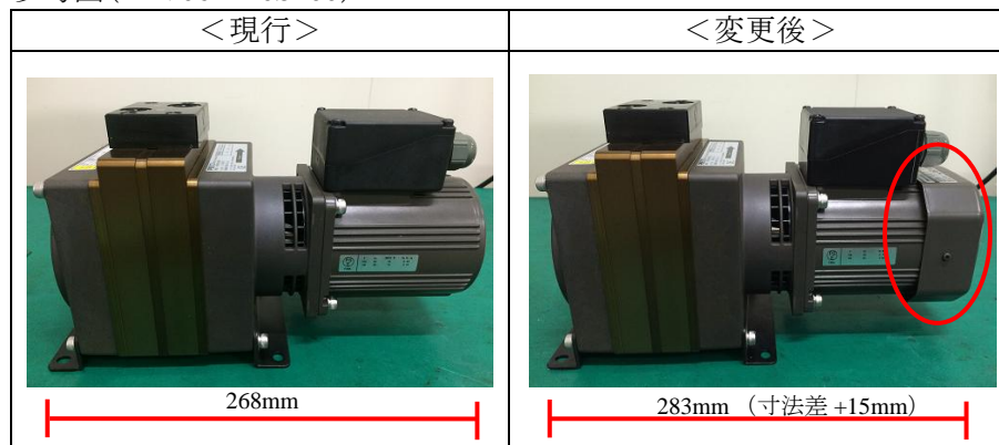
参考図 (RPV06A-40S100)
