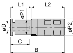
開放リング ミニタイプ \phi D : 4~6
