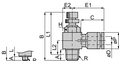
メートルネジタイプ
