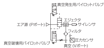
本ページ共通回路図
