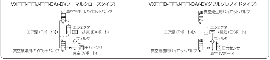
本ページ共通回路図
