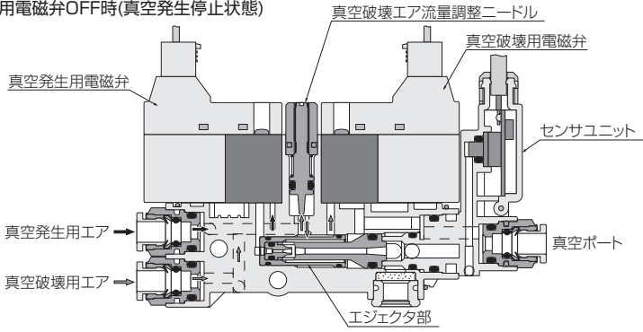
②.真空発生用電磁弁ON時(真空発生状態)
