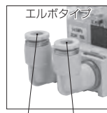
真空発生用 エア供給ポート
