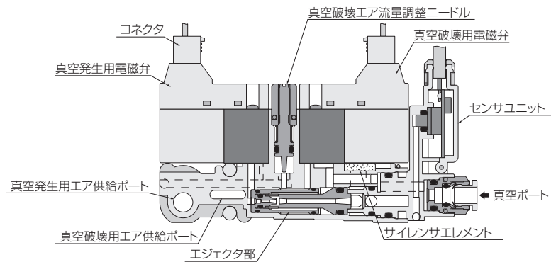
マニホールドタイプ 圧力センサ付
