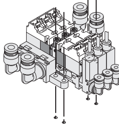
単体タイプにブラケットを使用し固定する場合
