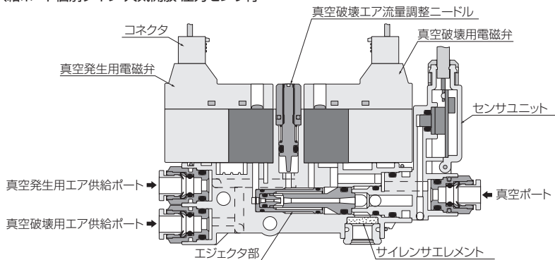
エア供給ポート個別タイプ 大気開放 圧力センサ付
