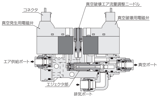
エア供給ポート共通タイプ 集中排気 圧力センサ無し
