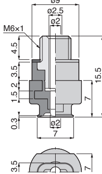
VP3.5x7[5]-M6[9] 質量：1.9g[2.1g]
