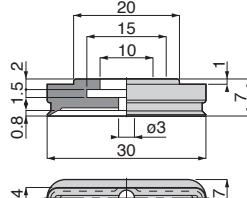
VP4×30E ⑤ 質量：1.1g
