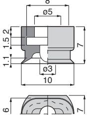
VP6×10E ⑤ 質量：0.4g[0.5g]
