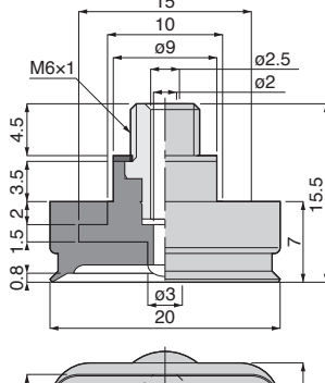
VP5x20E[5]-M6[9] 質量：2.4g[2.8g]
