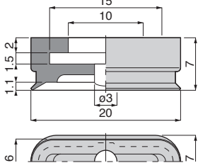
VP8×20E ⑤ 質量：0.7g[1.1g]
