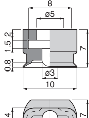
VP5×10E ⑤ 質量：0.3g[0.5g]
