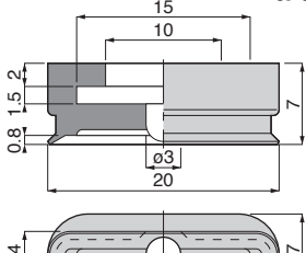
VP5×20E ⑤ 質量：0.7g[1.1g]
