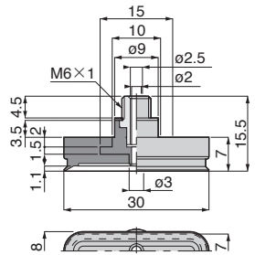
VP8×30E[5]-M6[9] 質量：2.9g[3.7g]
