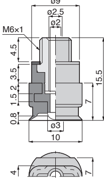
VP4x10E[5]-M6[9] 質量：1.9g[2.1g]
