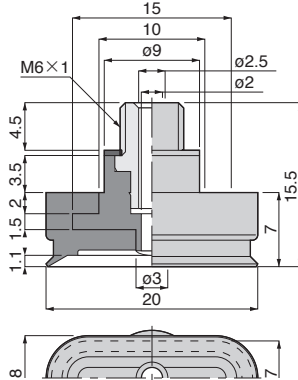
VP8×20E[5]-M6[9] 質量：2.5g[2.9g]
