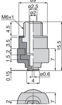
VP2x4E[5]-M6[9] 質量：1.9g[2.1g]
