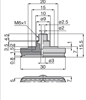
VP5x30E[5]-M6[9] 質量：2.8g[3.4g]
