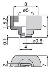
VP4×10E ⑤ 質量：0.4g[0.5g]
