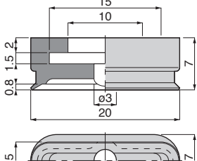
VP6×20E ⑤ 質量：0.7g[1g]
