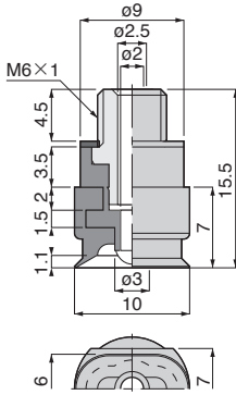
VP6×10E[5]-M6[9] 質量：1.9g[2.1g]
