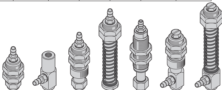
VPA VPMA バーブ継手 VPB VPMB バーブ継手 VPC VPMC バーブ継手 VPOC バーブ継手 VPLFC バーブ継手 VPD VPMD バーブ継手 VPOD バーブ継手
