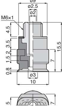
VP5x10E[5]-M6[9] 質量：1.9g[2.1g]
