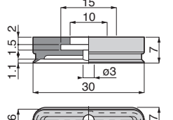
VP6×30E ⑤ 質量：1.2g[1.9g]
