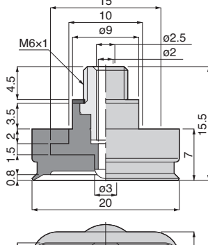
VP4x20E[5]-M6[9] 質量：2.4g[2.8g]
