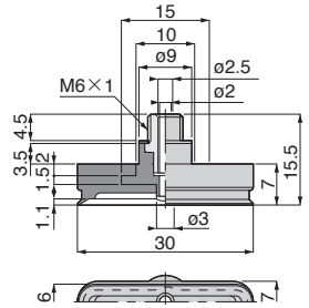
VP6×30E[5]-M6[9] 質量：2.9g[3.6g]
