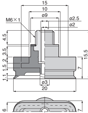
VP6×20E[5]-M6[9] 質量：2.4g[2.8g]
