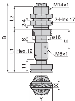
VPD 2 3 E 5 -M6 9
