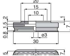
VP5×30E ⑤ 質量：1.1g[1.7g]
