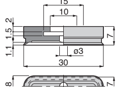
VP8×30E ⑤ 質量：1.2g[1.9g]
