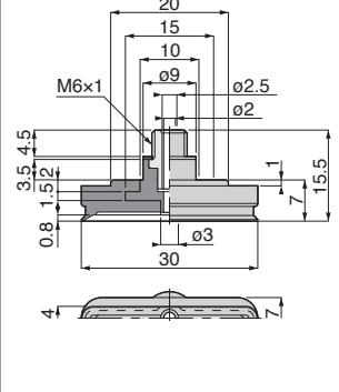
VP4x30E[5]-M6[9] 質量：2.8g[3.5g]
