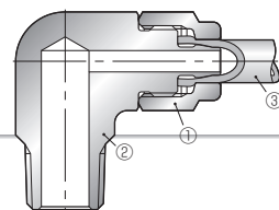
图为 L 型弯头：NSL
