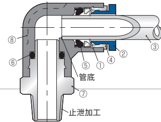
图为 L 型弯头：PL-SUS
