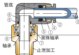
图为 L 型弯头：RL
