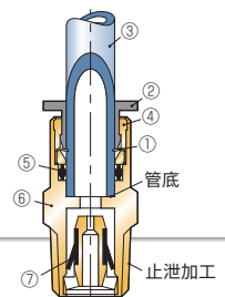
图为直通接头: JKC \phi 4 , \phi 6 mm
