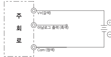
아날로그 출력의 배선(예)
